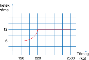
Quick-lift szivattyú diagram
